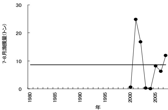
図3 播磨灘東部（兵庫県側：左上）、播磨灘南西部（香川県側：右上、平年値は1989～2007年の平均値）の標本漁協のシラス漁獲量、および播磨灘北西部（岡山県側：左下）の標本船のシラス漁獲量（実線は平年値）
